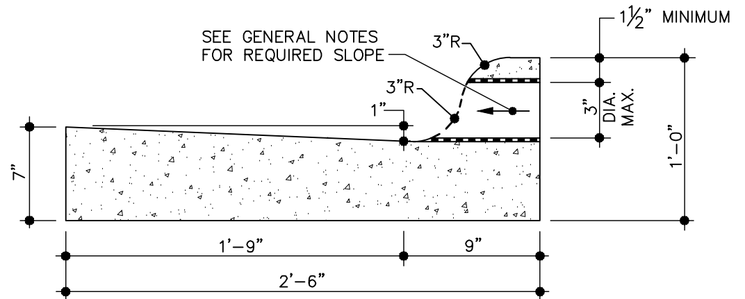
SECTION A-A
