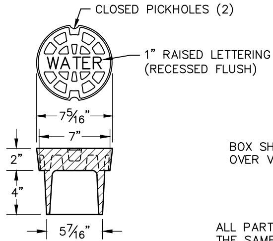
LID
