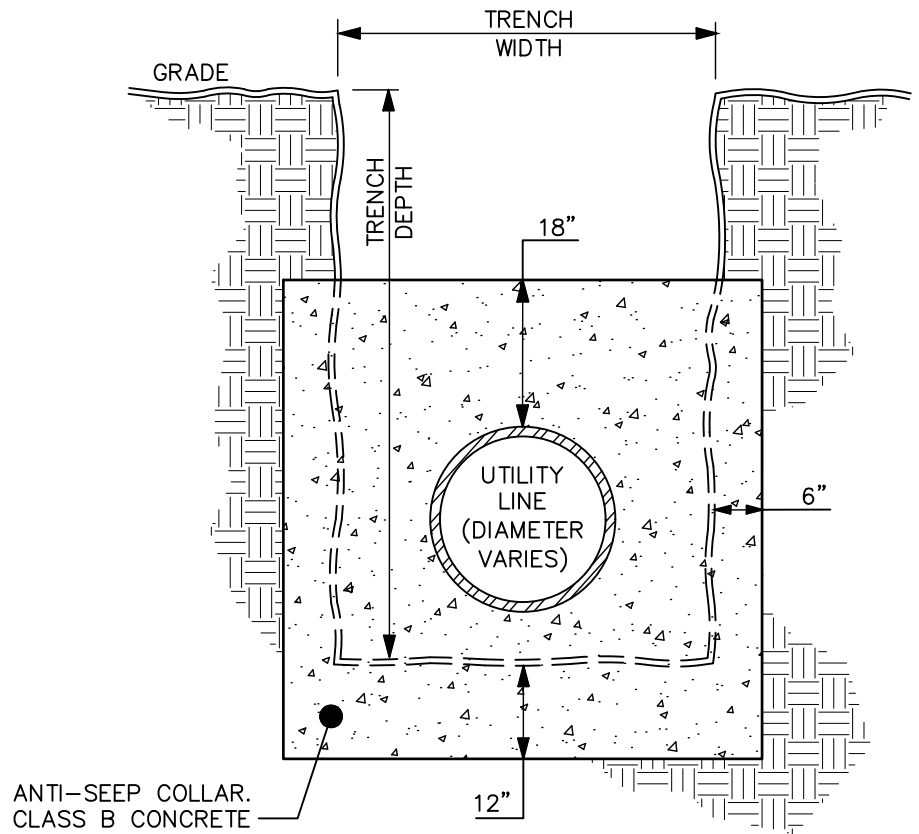
SECTION A-A
